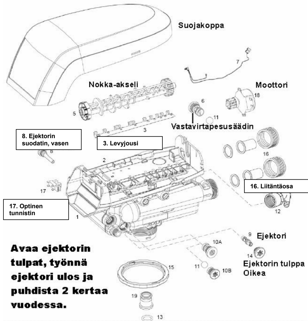
Kuva: Keskusventtiiliyksikönrakennetta
