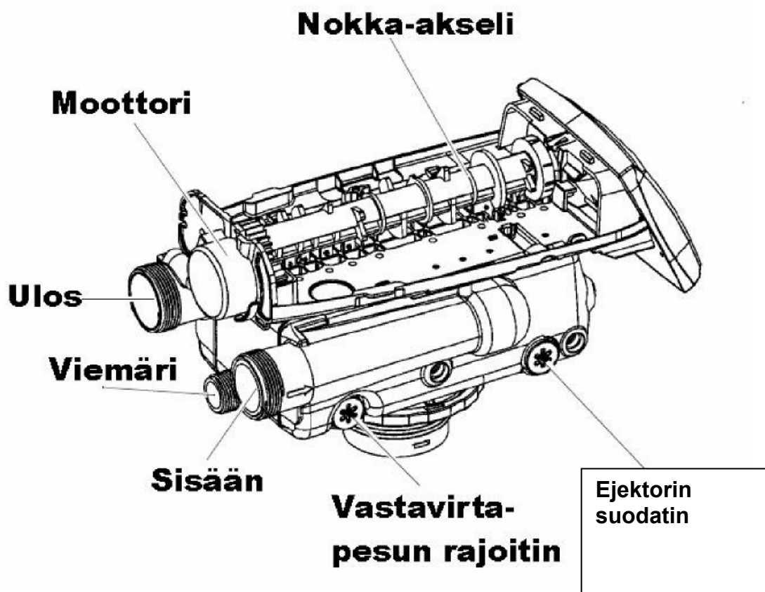
Kuva: Keskusventtiiliyksikön rakennetta 2
