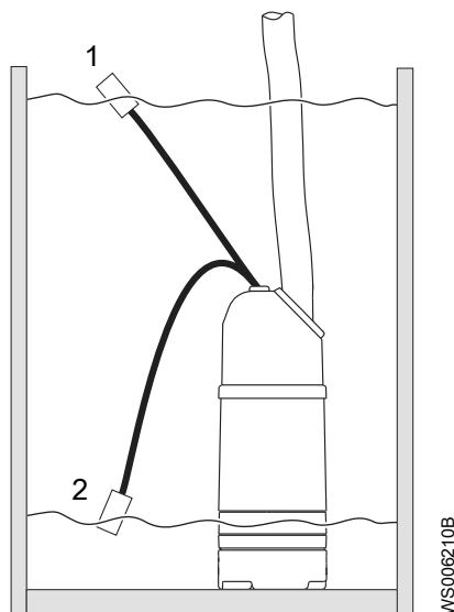
Kuva 1: Pintavipan toiminnot
